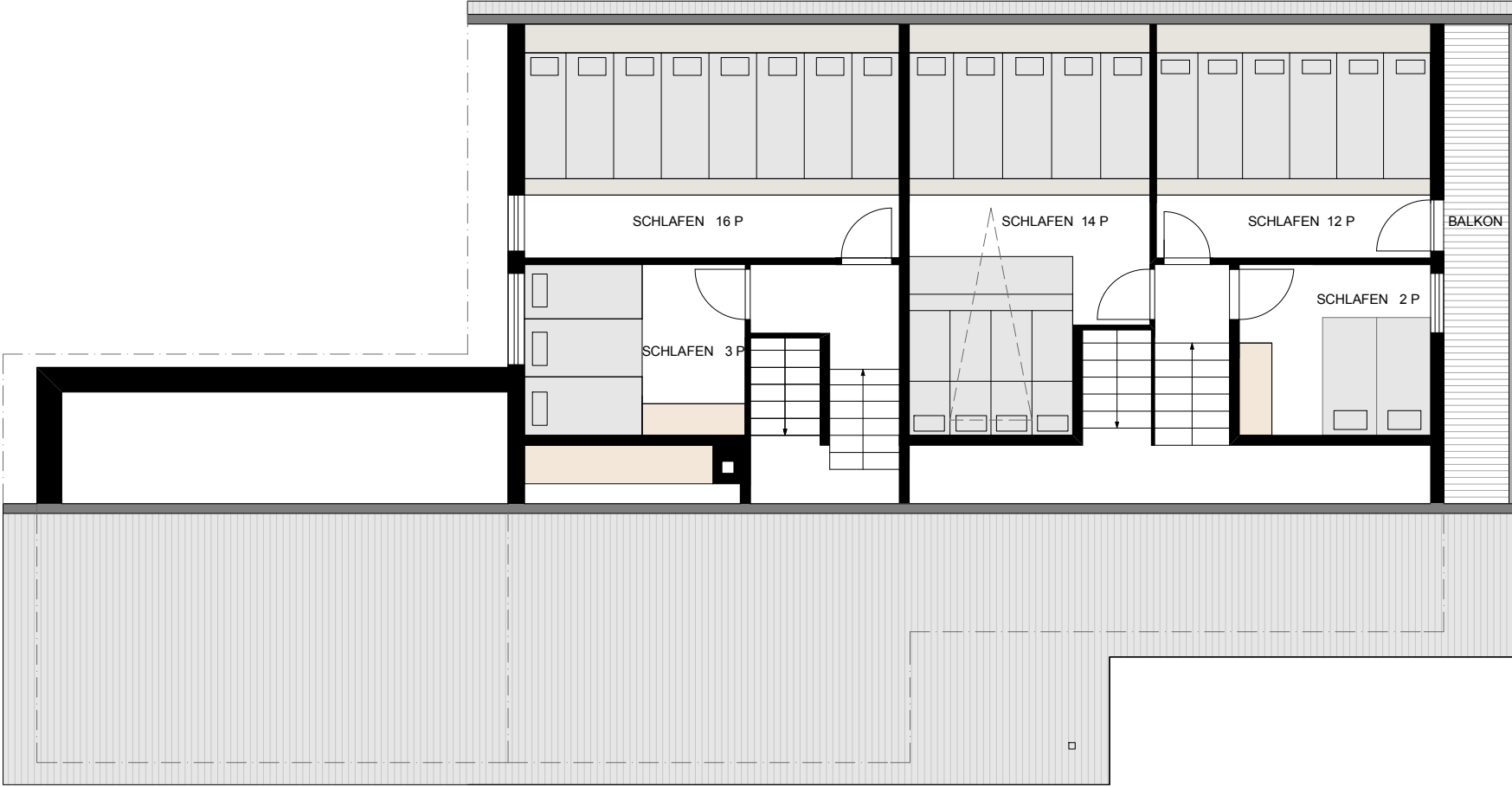
Grundriss Obergeschoss
